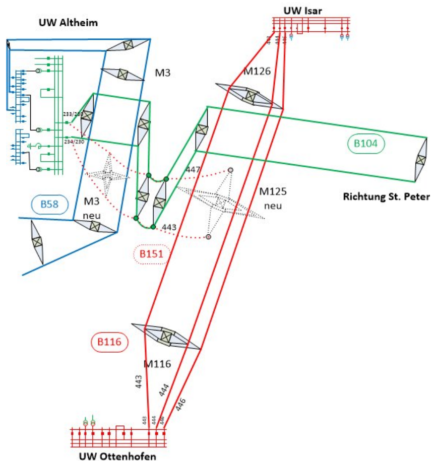
Abbildung 2: Errichtung der Masten zwischen UW Altheim bis Einbindung B116
