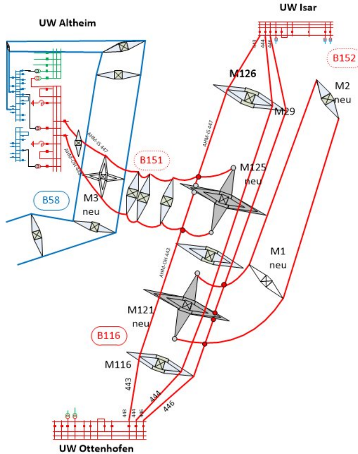
Abbildung 7: Abschluss Spannungsumstellung auf 380-kV zwischen Alheim und Adlkofen und Rückbau Bestandsmasten 22 bis 25
