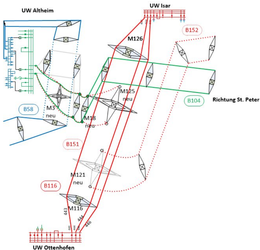
Abbildung 3: Inbetriebnahme des Abschnitts Altheim – Adlkofen auf 220-kV
