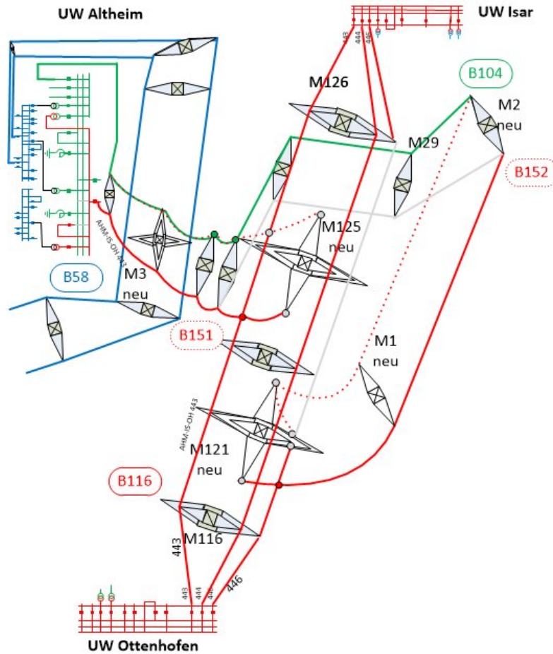
Abbildung 5: Beginn Spannungsumstellung auf 380-kV zwischen Altheim und Adlkofen
