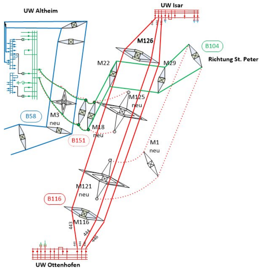
Abbildung 4: Rückbau zwischen Altheim und Adlkofen bis einschließlich Mast 21
