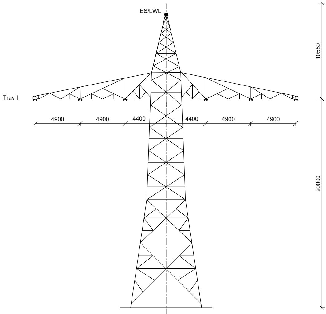
WEWA100-20,00 B57: Mast Nr. 5N
