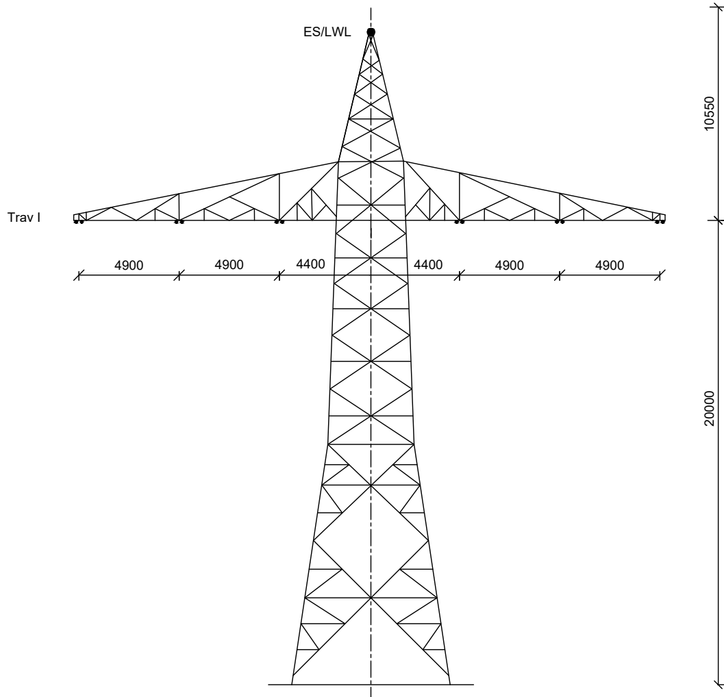
WEWA100-20,00 B58: Mast Nr. 1N
