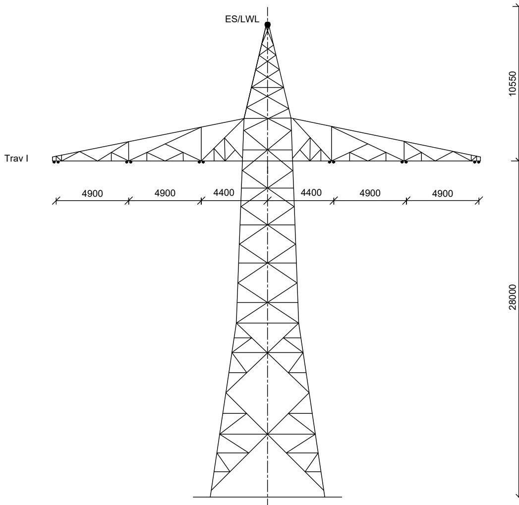
WEWA100-28,00 B57: Mast Nr. 21N
