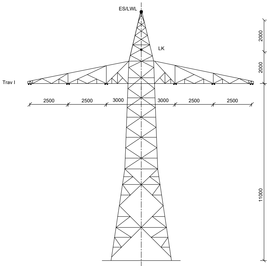
WE/WAdiff/120-11.00 B175A: Mast Nr. 1
