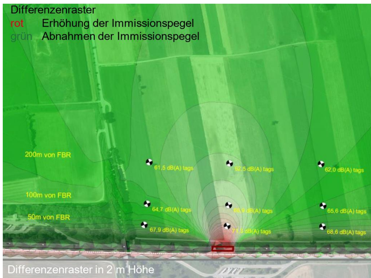
Abbildung 1 – Baulärmberechnung mit Änderung der Immissionspegel im Bereich lärmintensiver Tätigkeiten. Quelle: Autobahndirektion Südbayern
