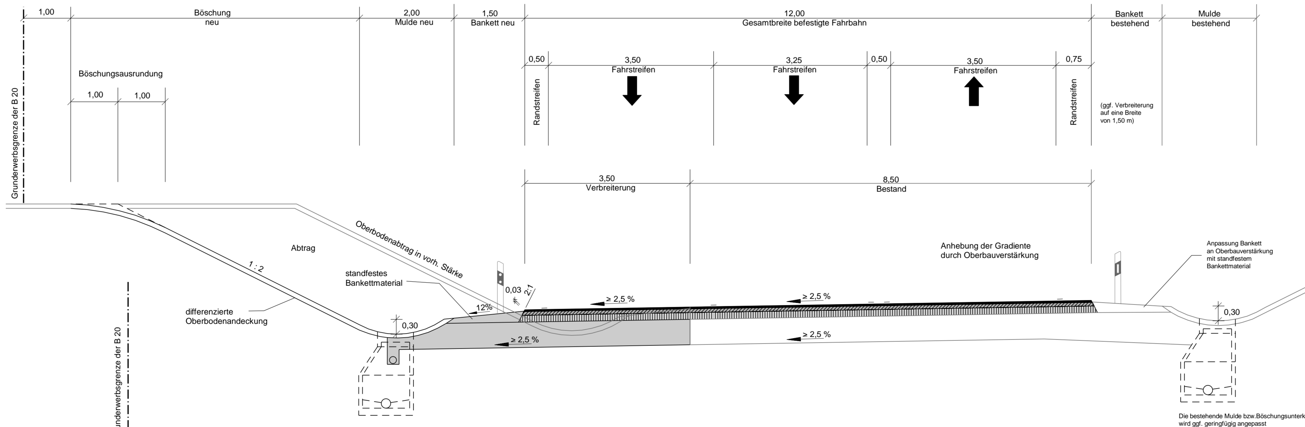
Oberbau mit lärminderndem Belag nach RLS 90
